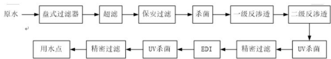
图 3.3-1 DI 水制备工艺流程图
