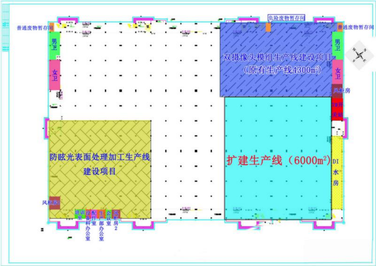
图 3.2-1 31 号厂房 1 楼平面布置
