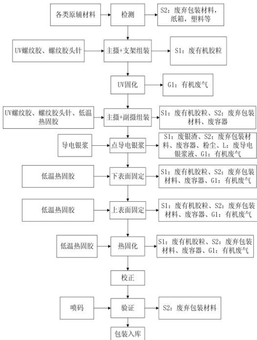
图 3.4-1 双摄像模组生产流程与产污环节示意图
