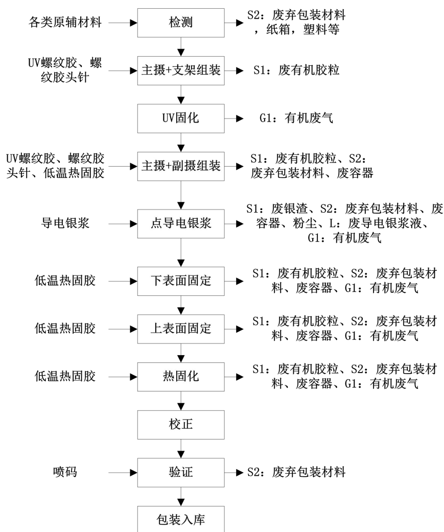
图 3.4-2 单摄像模组生产流程与产污环节示意图
